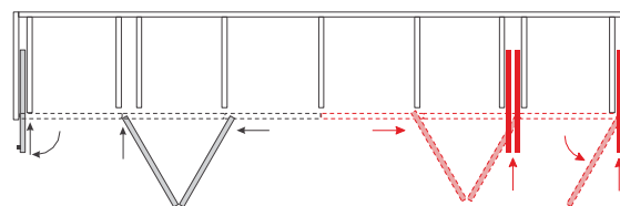
В комбинация HAWA-Concepta 25/30/40/50 and HAWA-Folding Concepta 25
