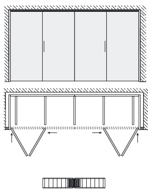
Монтаж без корпус
