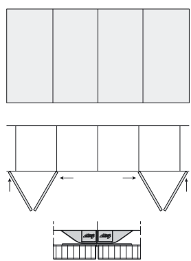
Пълно припокриване с долна релса
